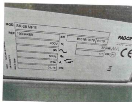
Uscator rufe profesional Fagor Nr.inventar 4
