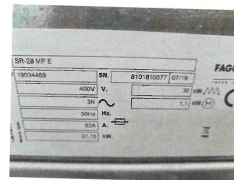
Uscator rufe profesional Fagor Nr.inventar 3
