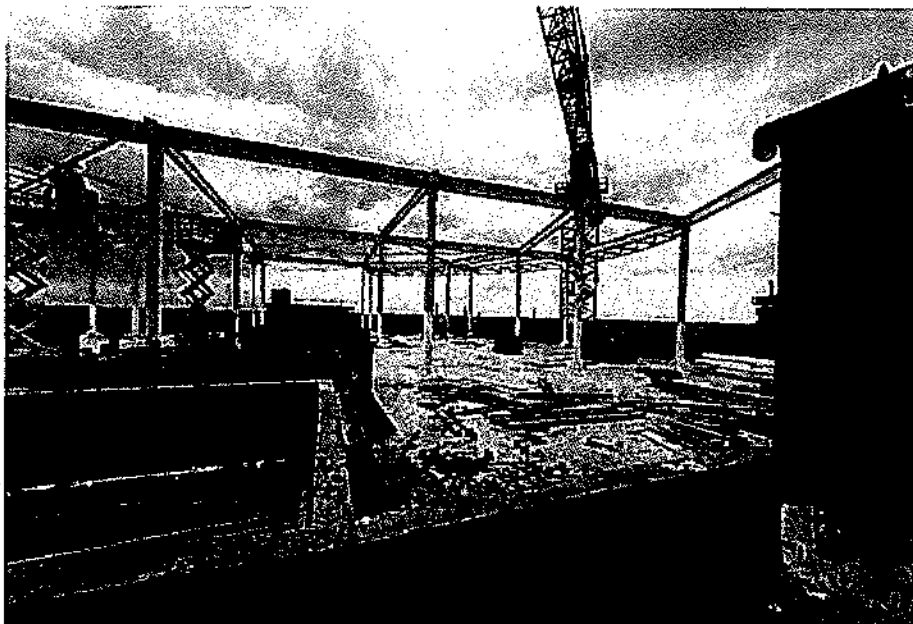
Figura 1.9. Executia lucrari de decofrare planseu peste etaj 7
